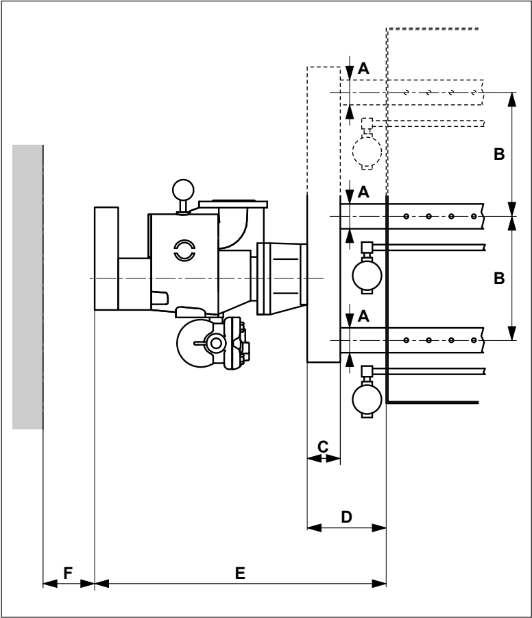
Masse für Doppel- und Dreifachrohre
