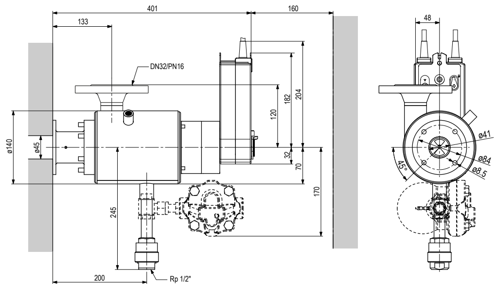
Antrieb CA150A / CA150A-S Condair Esco 10 Edelstahl-Ausführung
