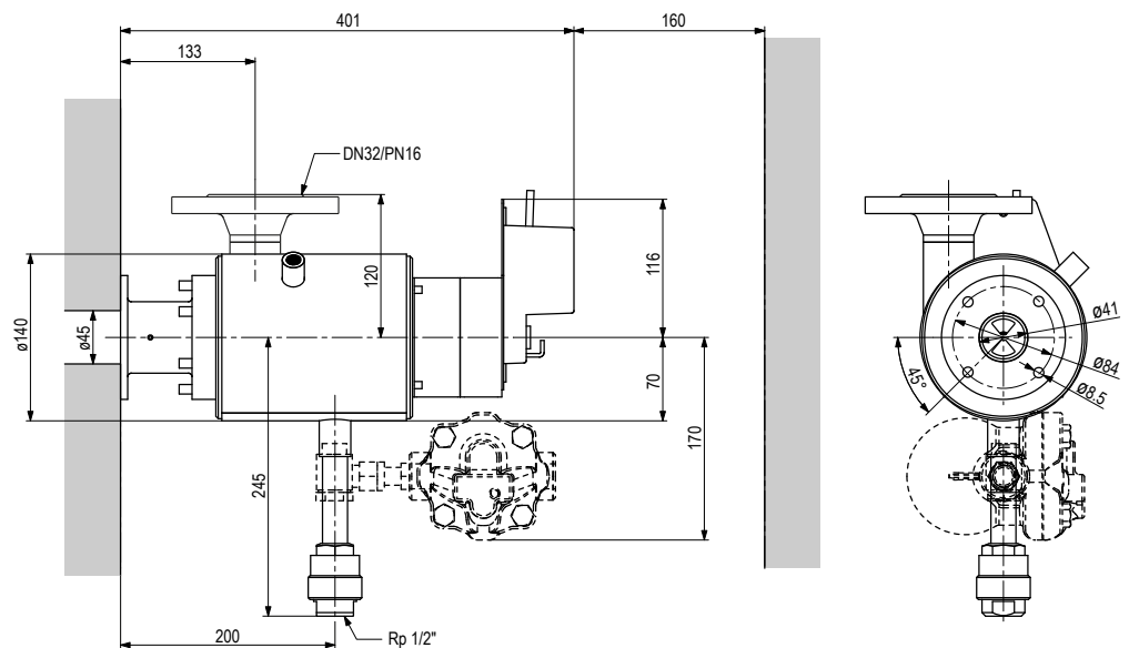
Antrieb CA75 Condair Esco 10 Edelstahl-Ausführung
