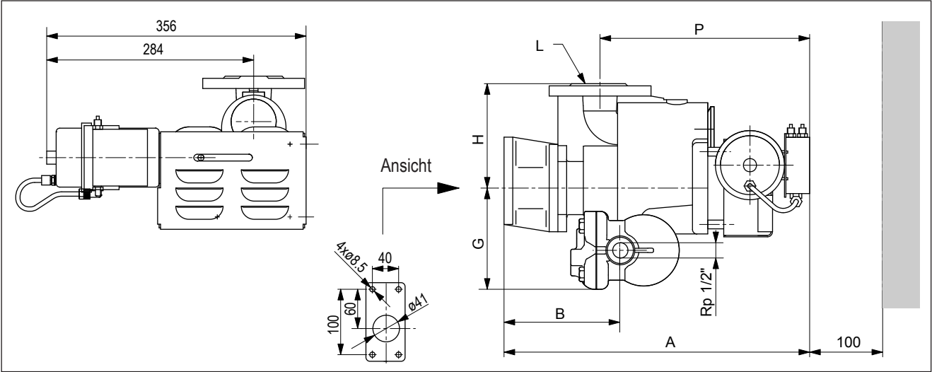
Condair Esco 20 und Condair Esco 30
