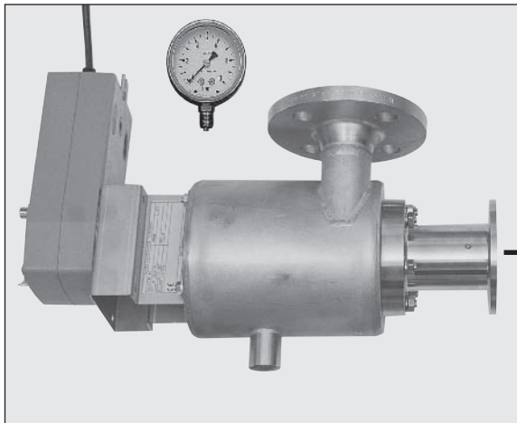
DR73 Registerverrohrung
