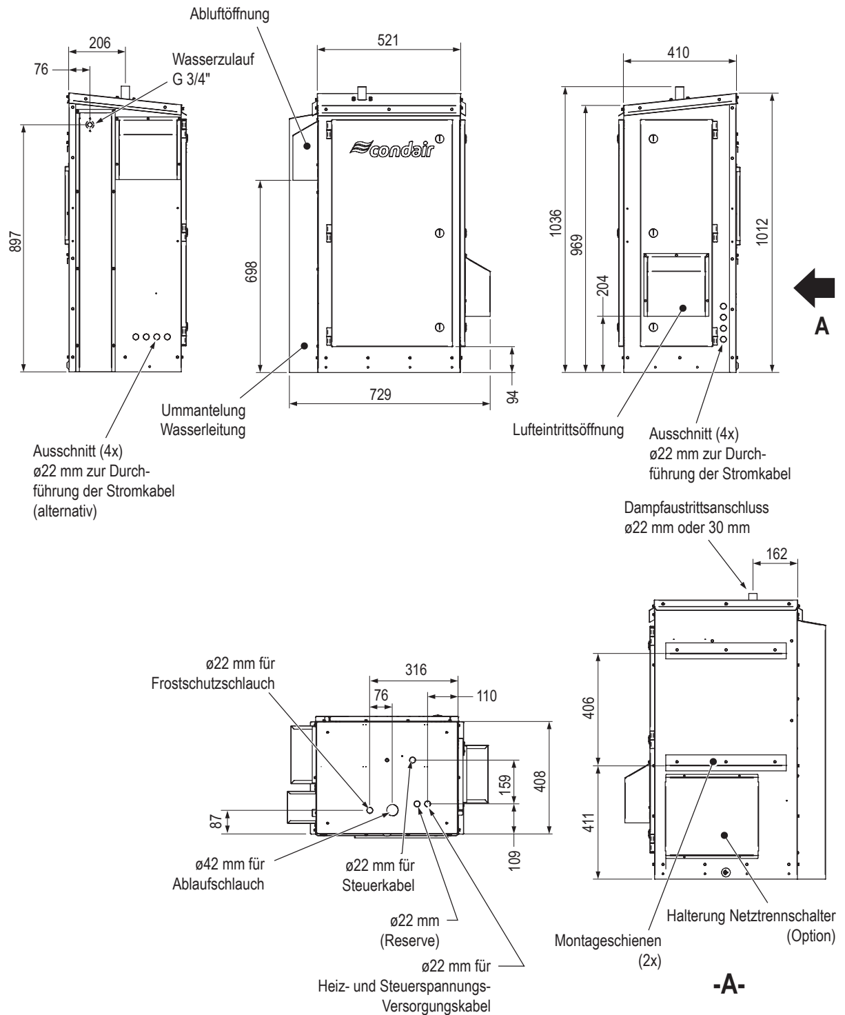
Abb. 24: Condeair EL/RS-Befeuchter für den Aussenbereich, kleines Gehäuse (EL-OC 5...15)
