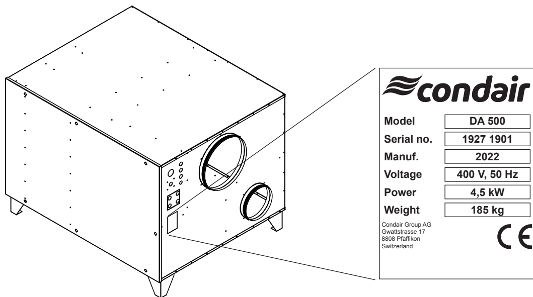
Abb. 1: Typenschild
