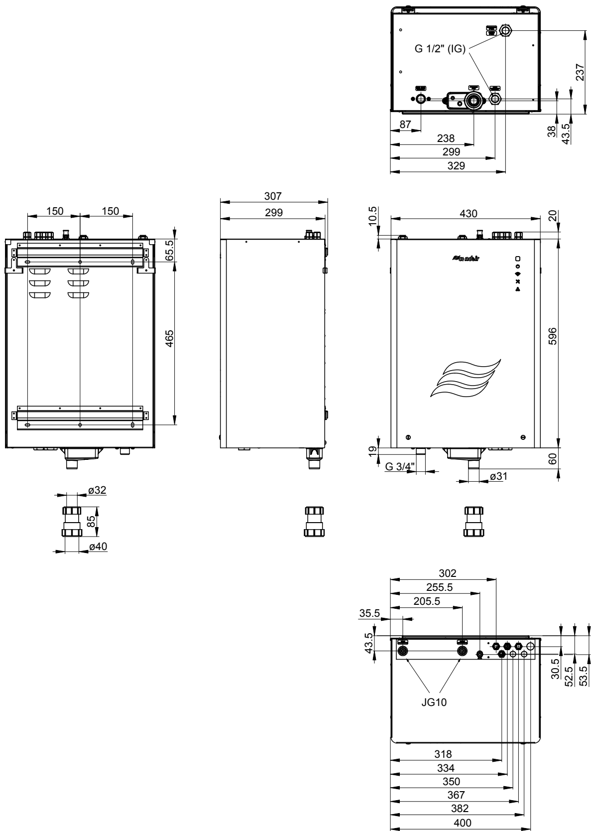
Abb. 31: Massabbildung Hydraulikeinheit (Masse in mm)
