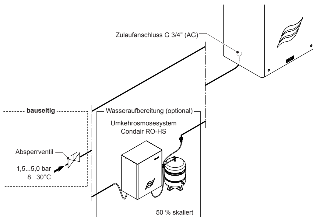
Abb. 18: Installation Frischwasserzulauf
