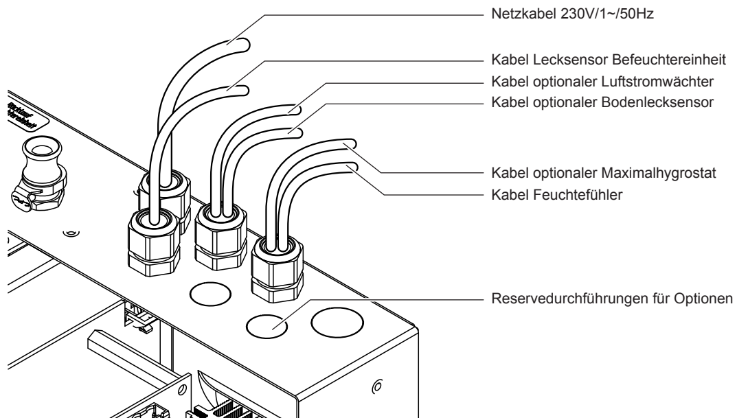
Abb. 26: Kabeleinführung
