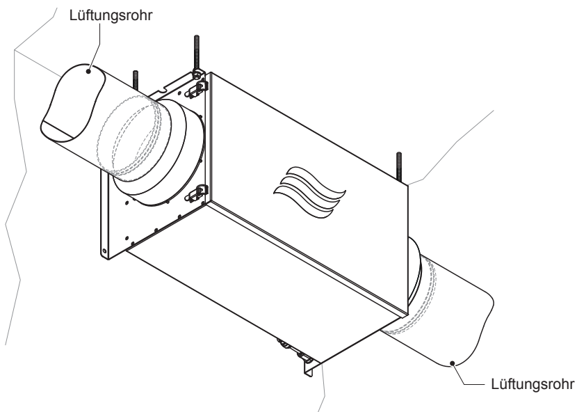
Abb. 10: Lüftungsrohre montieren
