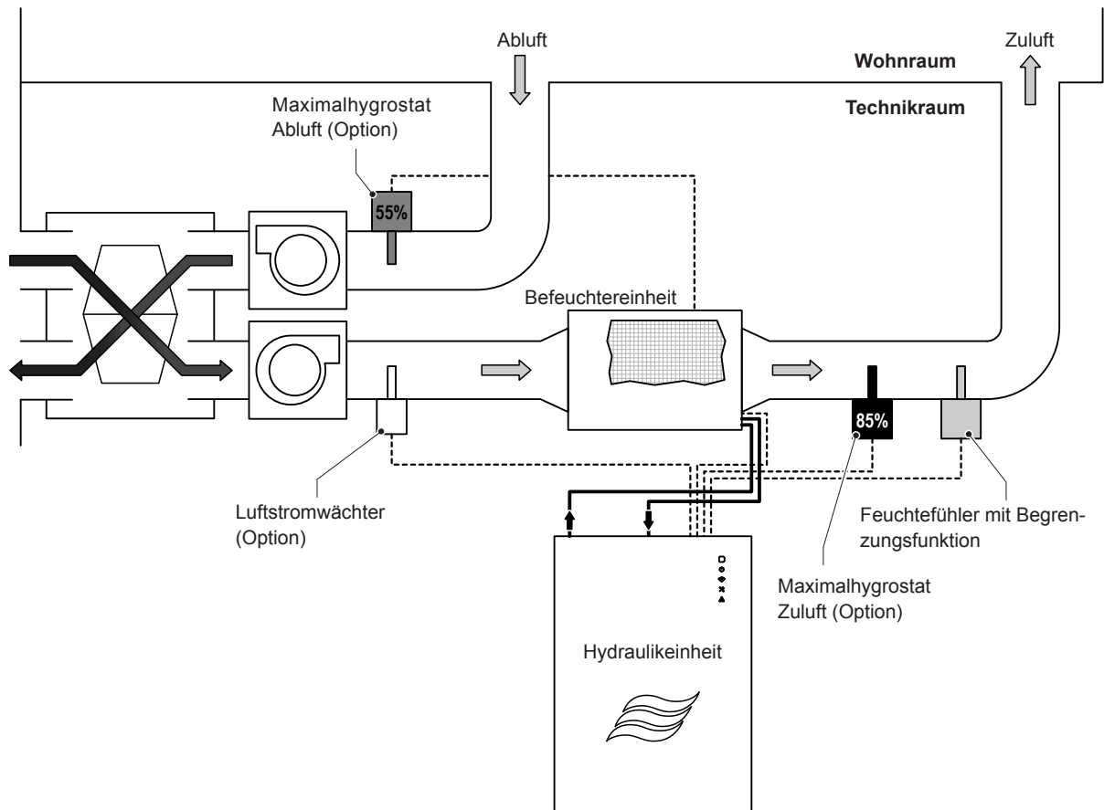
Abb. 21: Prinzipschema Zuluft-Feuchteregelung
