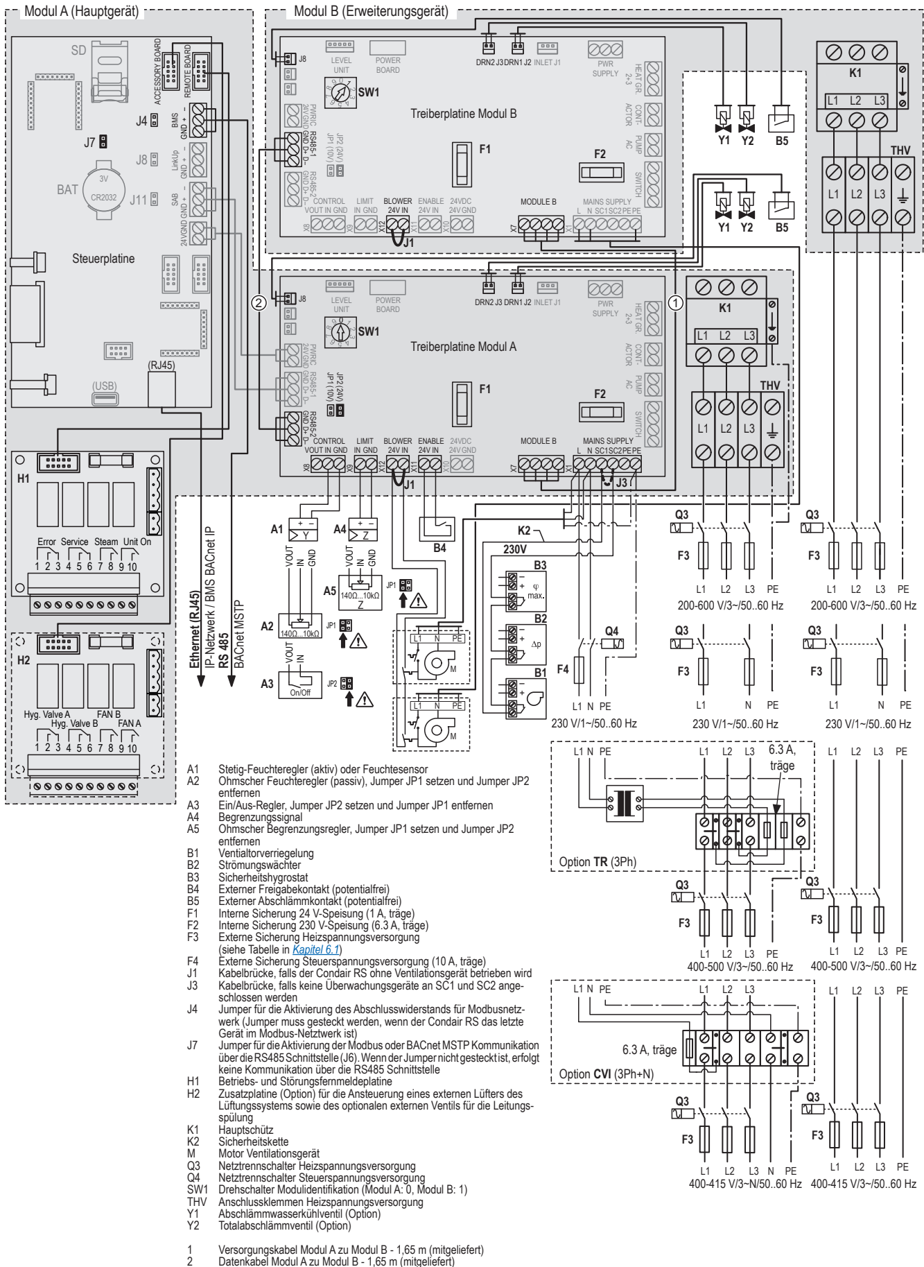
Abb. 26: Elektroschema Condair RS - Doppelgeräte (2 x Einzelgehäuse "M") 40...80 kg/h
