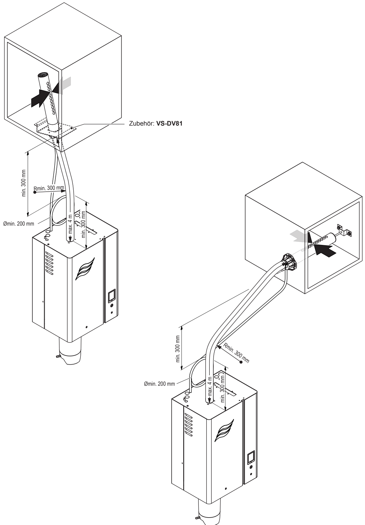
Abb. 15: Dampfverteilrohr ist mehr als 500 mm über der Geräteoberkante montiert
