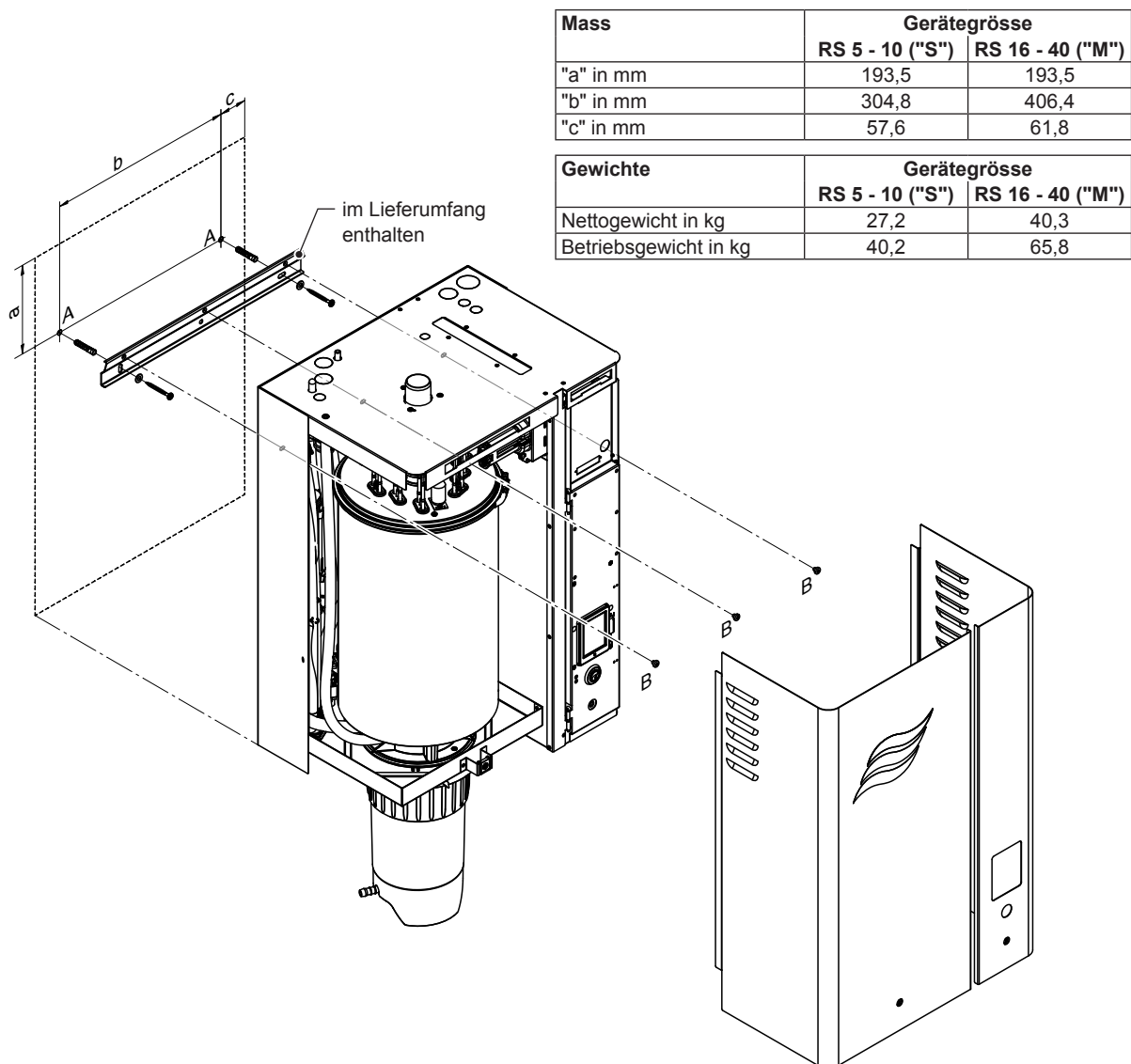
Abb. 10: Übersicht Montage von Einzelgeräten Klein und Mittel
