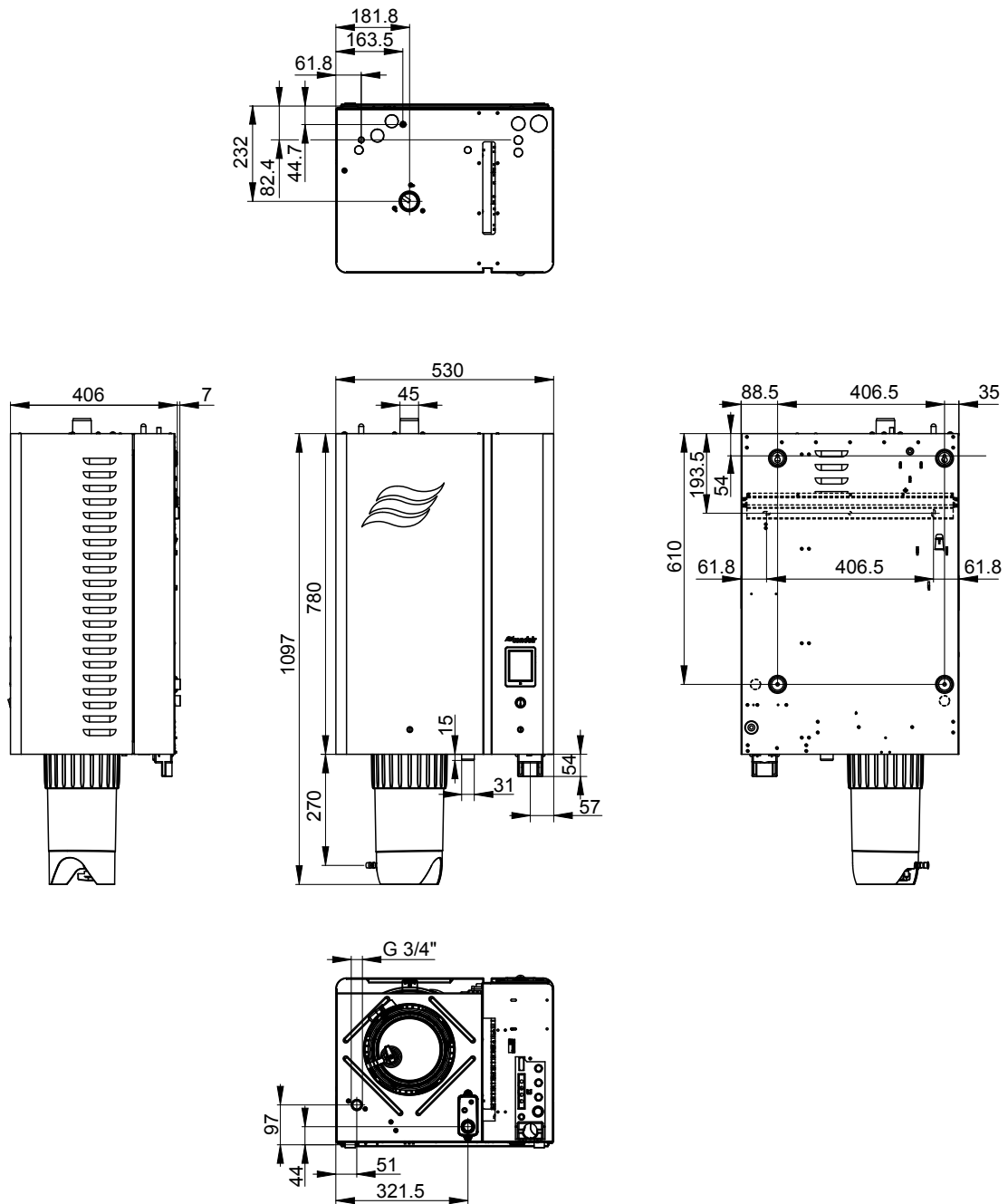
Abb. 29: Masszeichnung Gerät "M" (Masse in mm)
