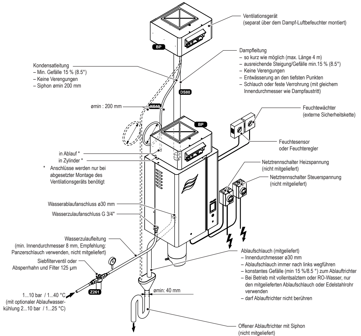
Abb. 8: Typische Installation für Direkt-Raumbefeuchtung
