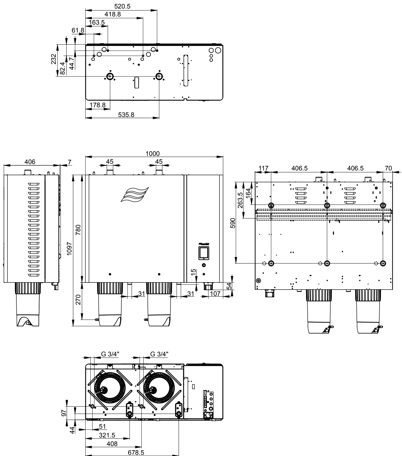
Abb. 30: Massabbildung Gerät "Large" (Masse in mm)
