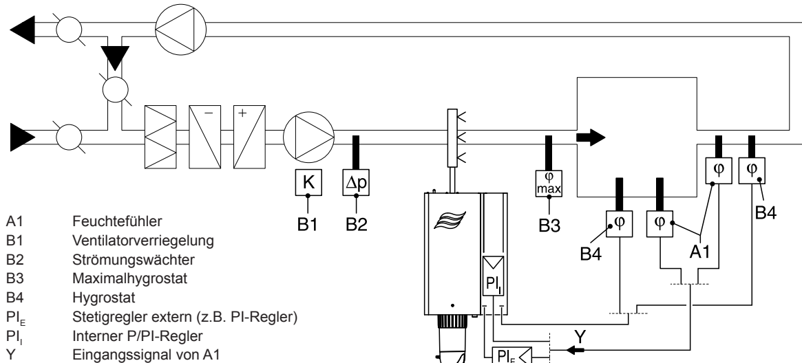
Abb. 21: System 1 – Raumfeuchteregelung
