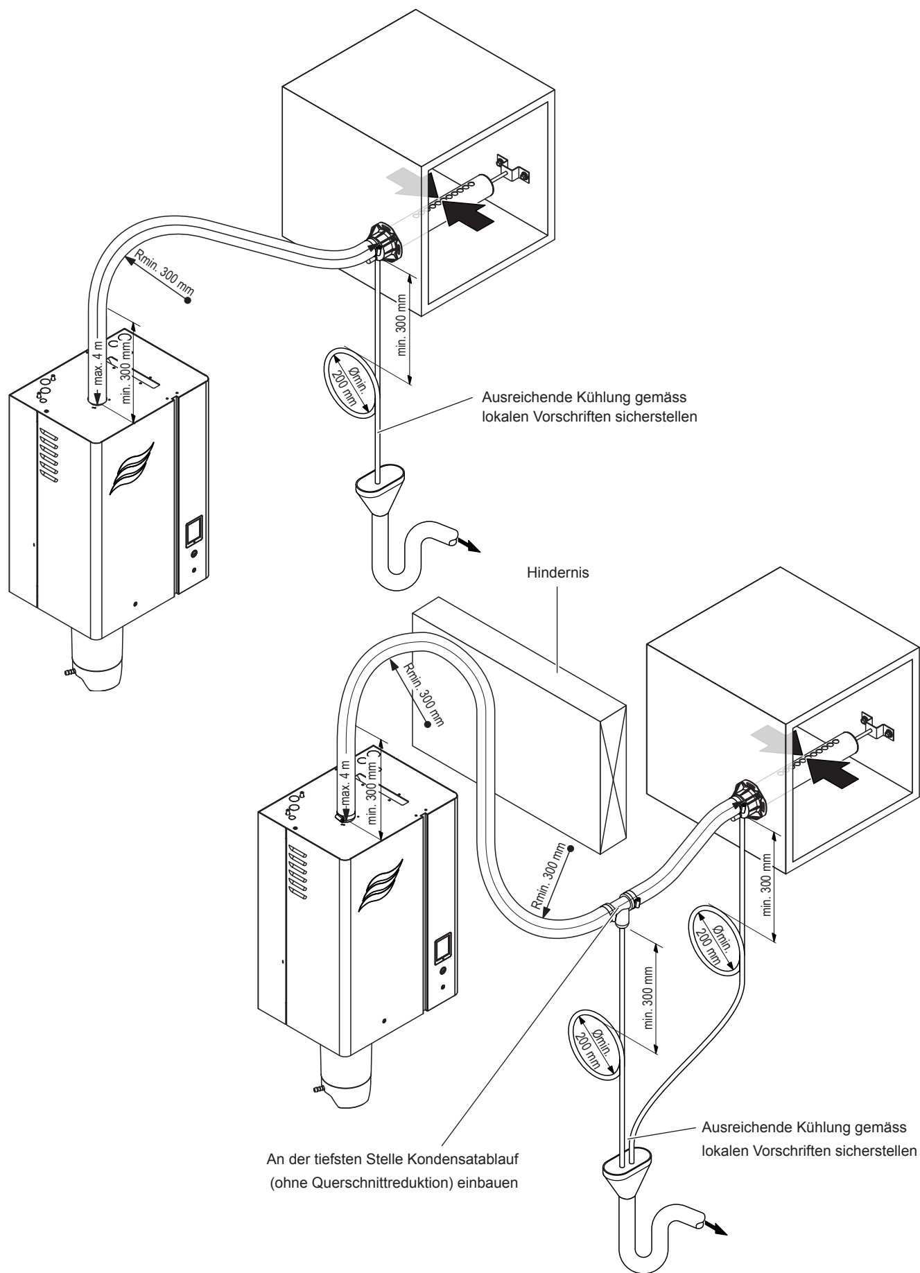
Abb. 16: Dampfverteillrohr ist weniger als 500 mm über oder unter der Geräteoberkante montiert
