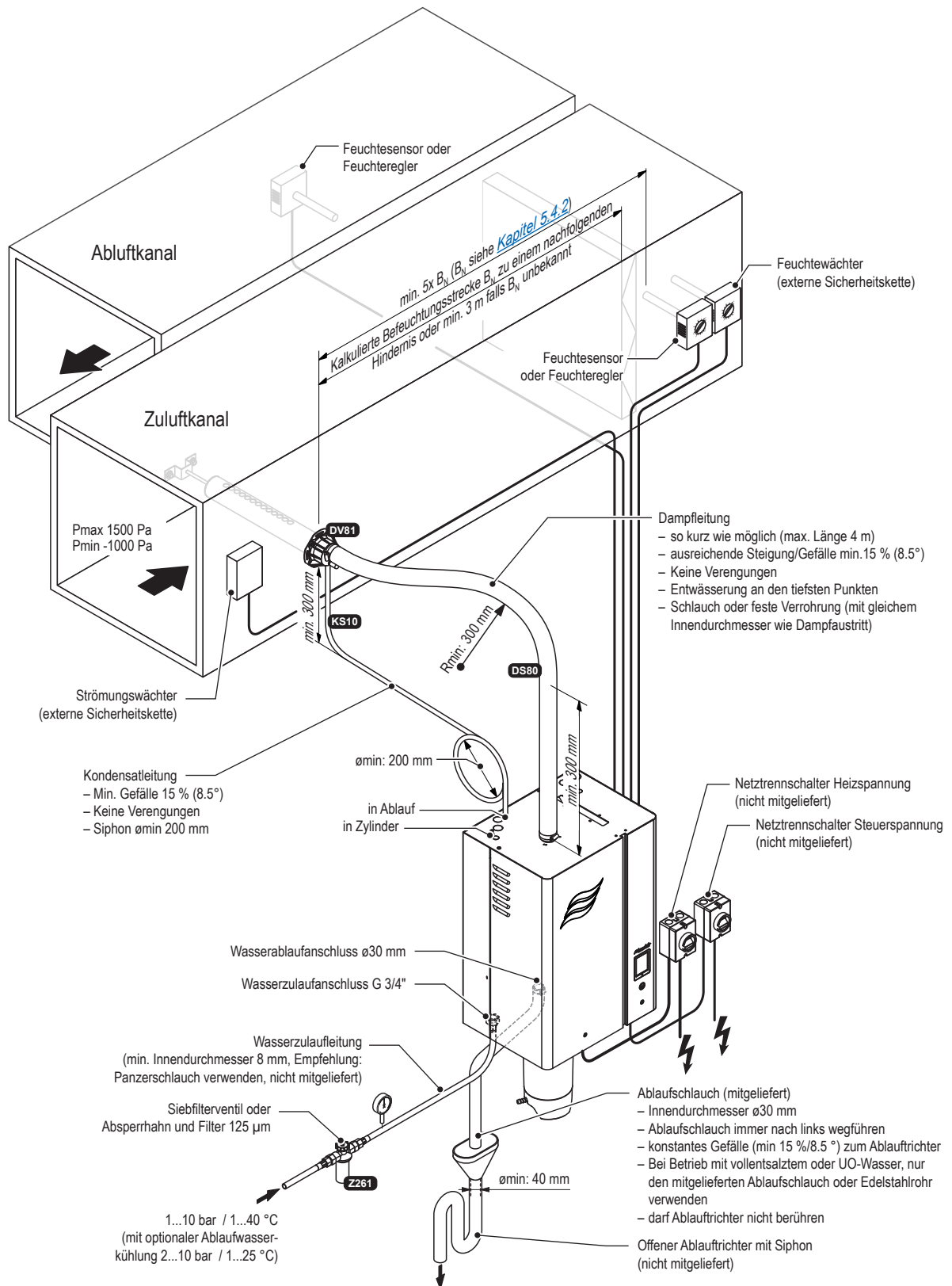
Abb. 7: Typische Installation für Kanalbefeuchtung
