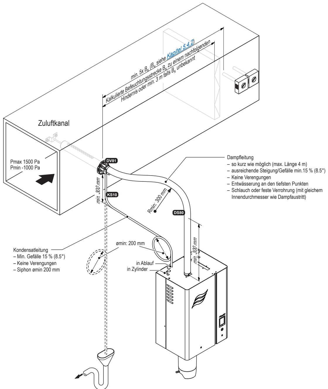
Abb. 12: Übersicht Dampfindallation Kanalluftbefeuchtung
