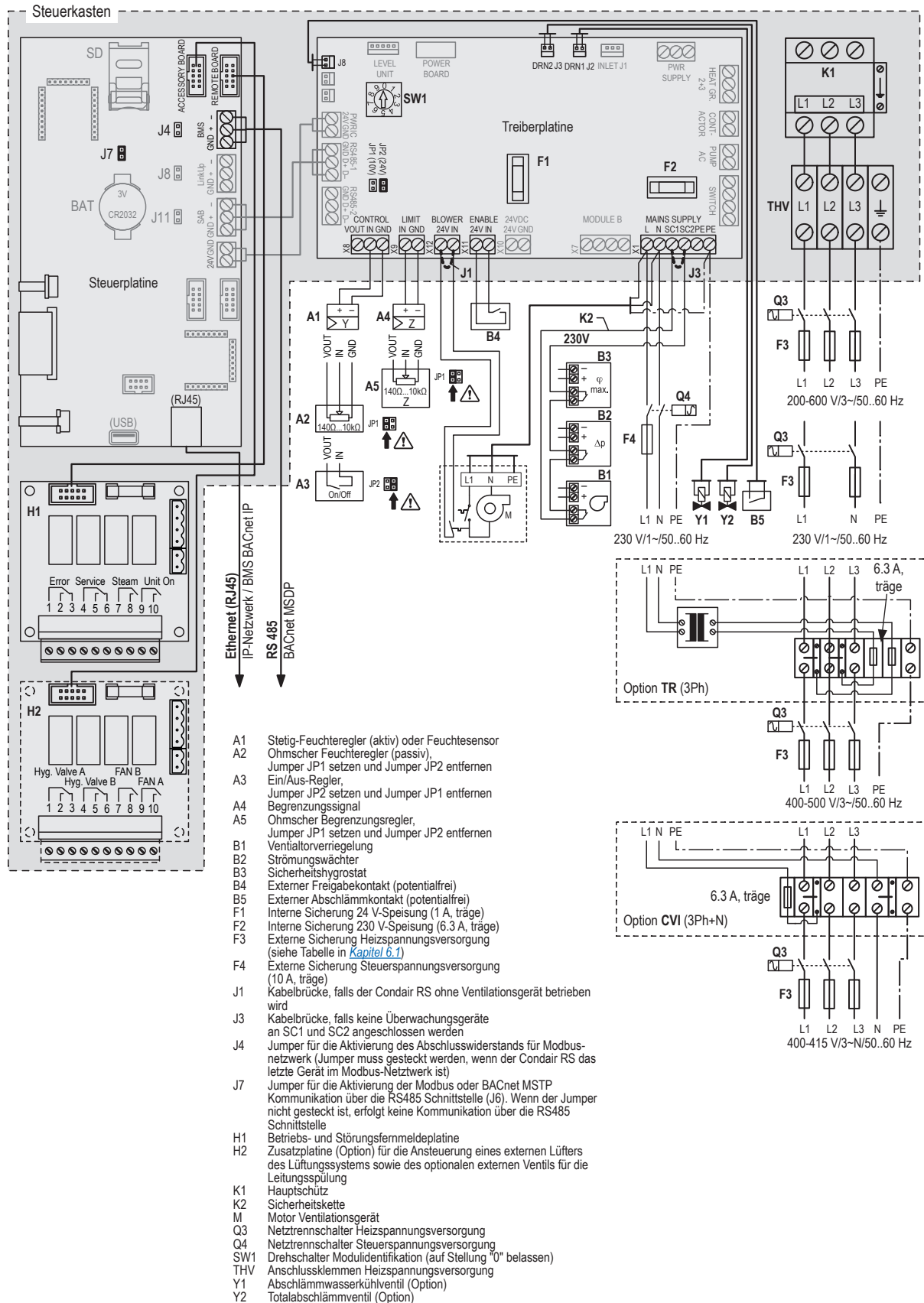
Abb. 24: Elektroschema Condair RS - Einzelgeräte "S" und "M" (5...40 kg/h)
