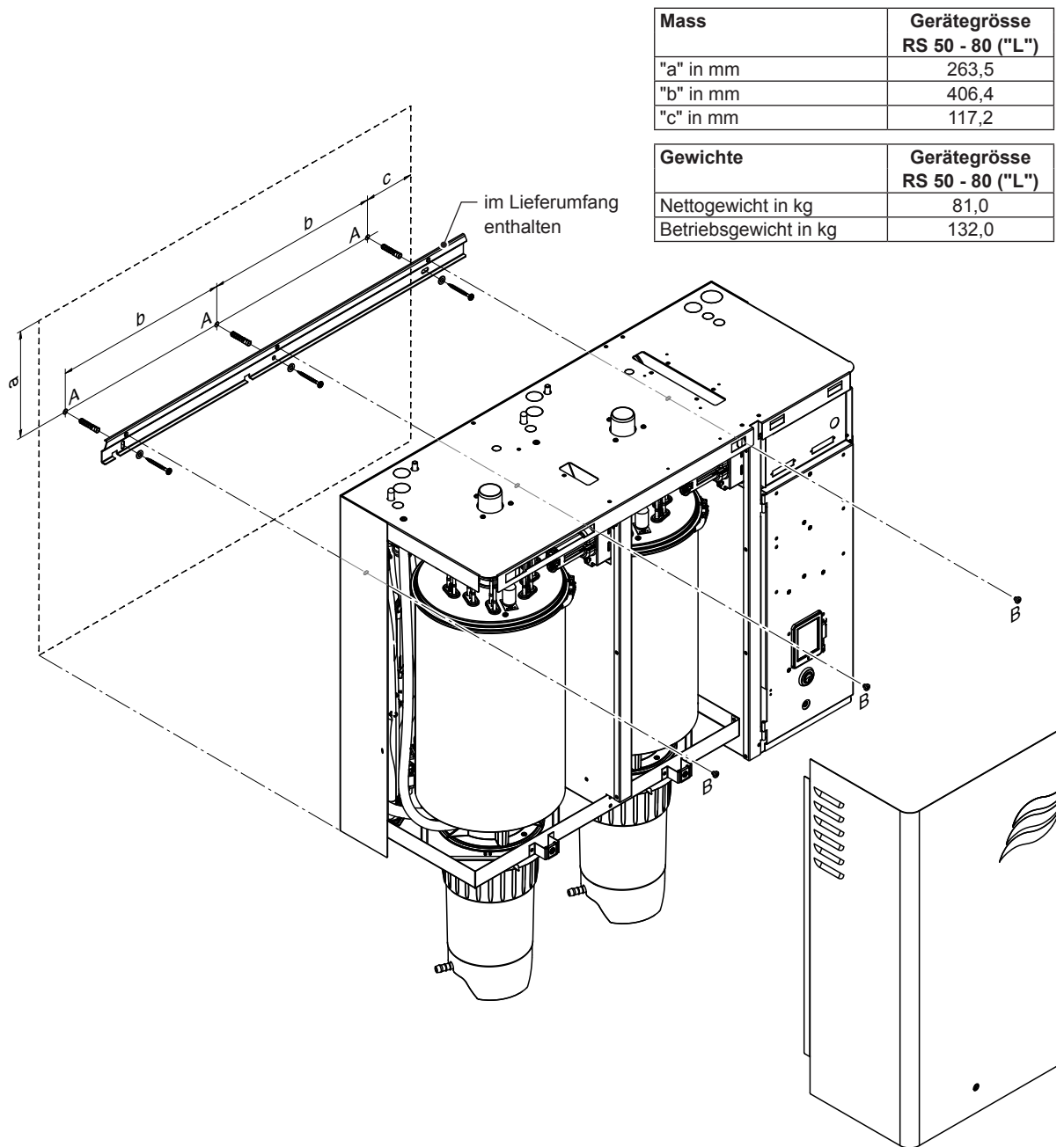
Abb. 11: Übersicht Montage von Einzelgeräten Gross
