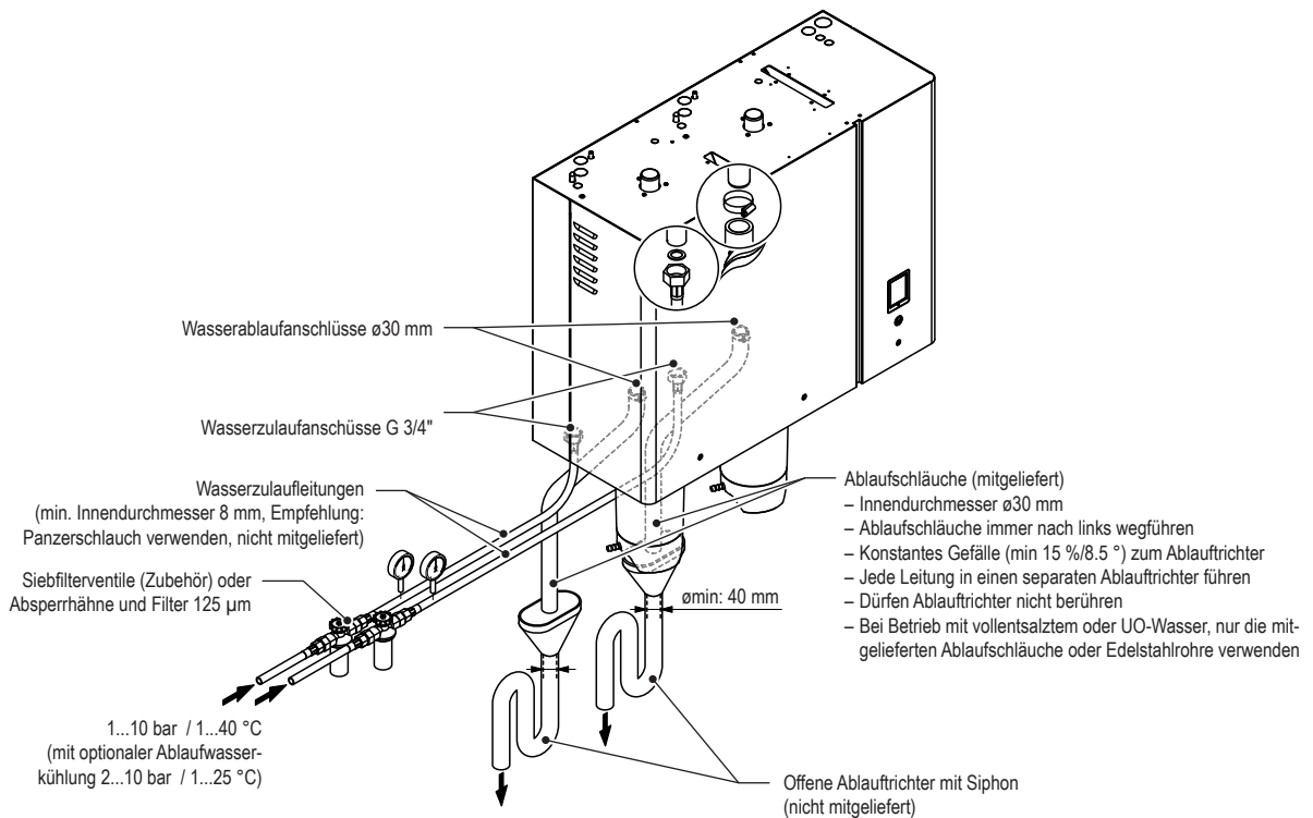
Abb. 20: Übersicht Wasserinstallation für Einzelgeräte Gross ("L")
