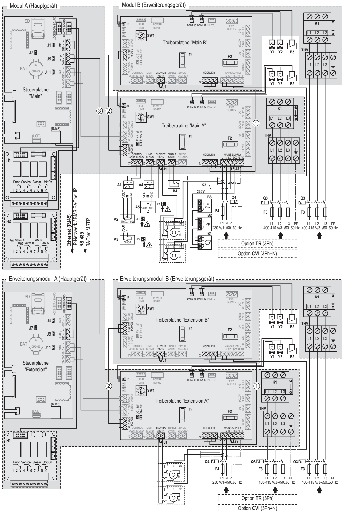
Abb. 27: Elektroschema Condair RS - Linkup-Systeme 100...160 kg/h
