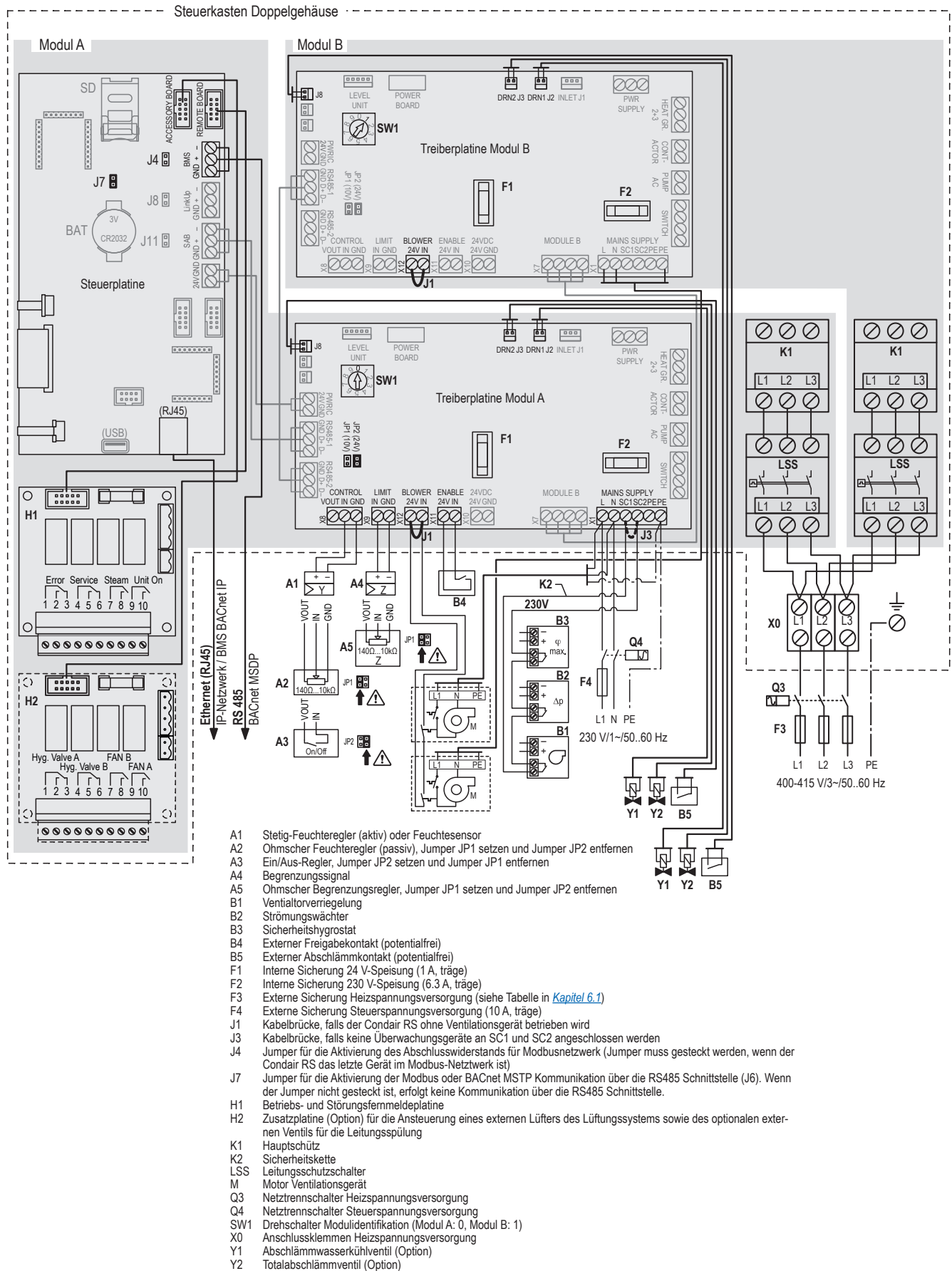
Abb. 25: Elektroschema Condair RS - Einzelgeräte "L" 50...80 kg/h
