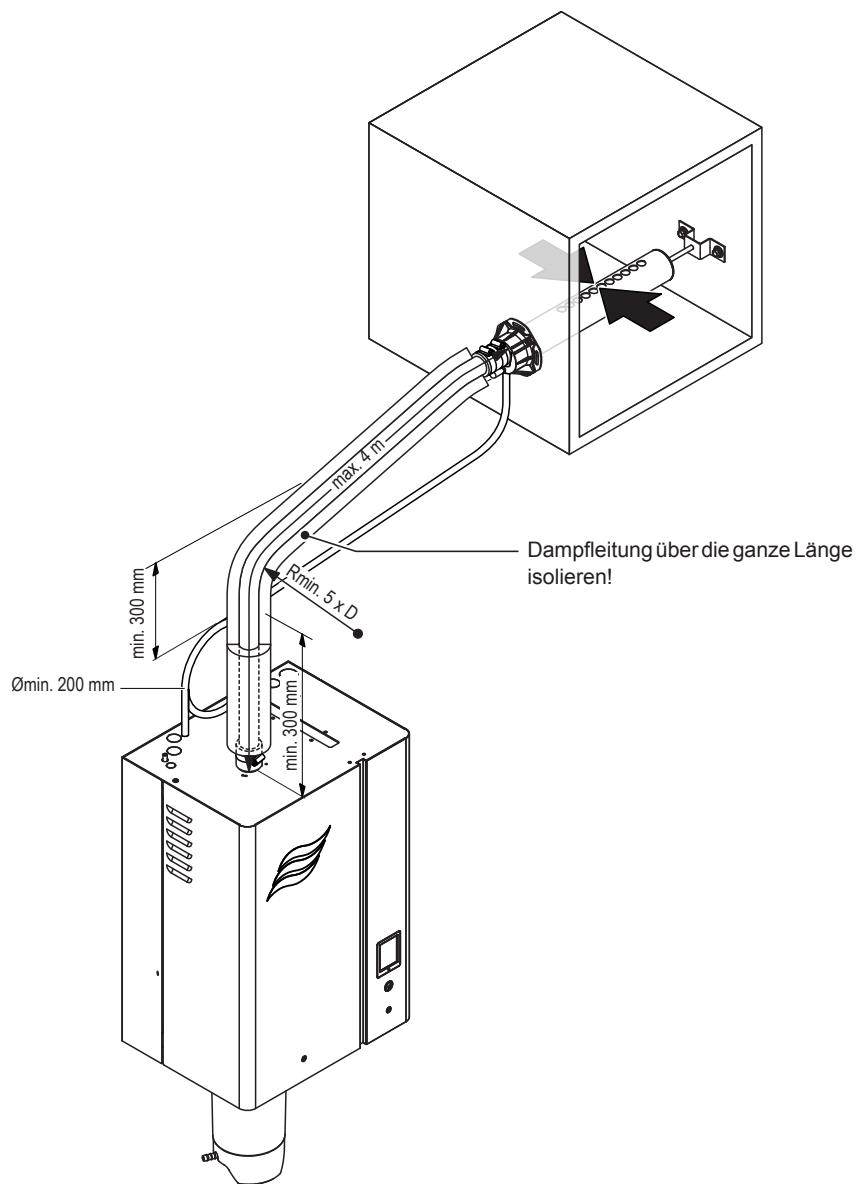
Abb. 17: Dampfleitung mit fester Verrohrung und Isolation
