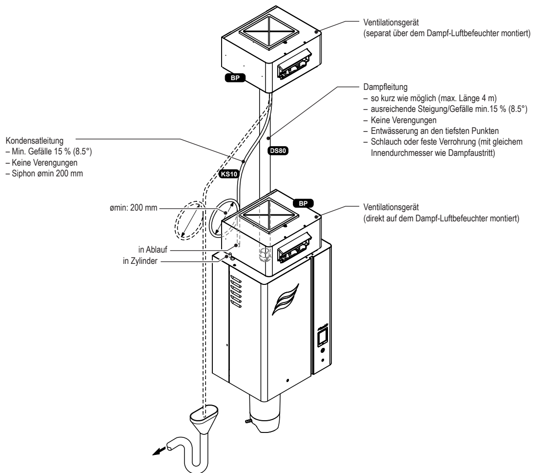
Abb. 13: Übersicht Dampfinstallation Direkt-Raumluftbefeuchtung
