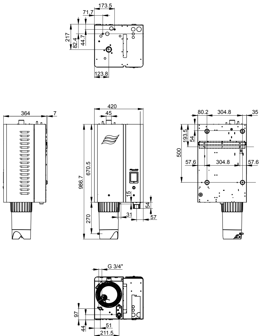
Abb. 28: Masszeichnung RS 5 - 10, Gehäusegrösse "S" (Masse in mm)
