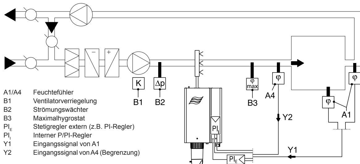
Abb. 22: System 2 – Raumfeuchteregelung mit stetiger Begrenzung der Zuluftfeuchte
