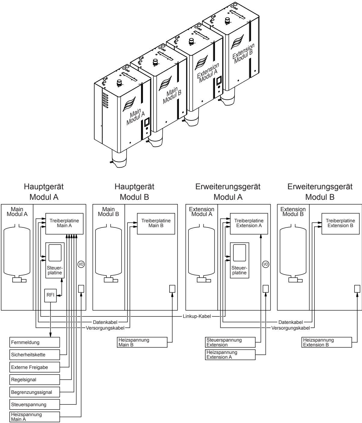
Abb. 5: Übersicht Linkup-Systeme (4 x "M")
