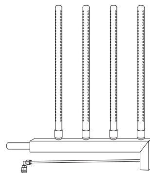
Baureihe DR 73 mit anlagenspezifischer Mehrfach-Verteilung
